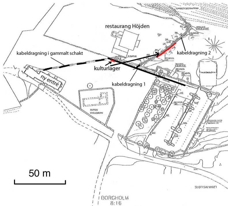
Figur 2. Kabeldragningen vid Borgholms slottsruin. Streckad linje = följer äldre kabelschakt, heldragen svart linje = kabeldragning 1, heldragen grå linje = kabeldragning 2, röd markering = observerat kulturlager.
