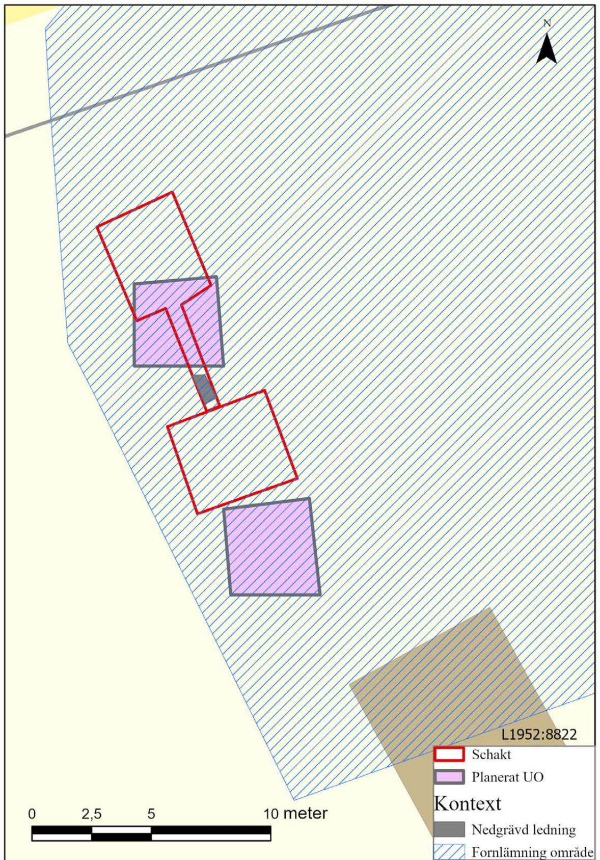
Figur 3 Schaktöversikt.
