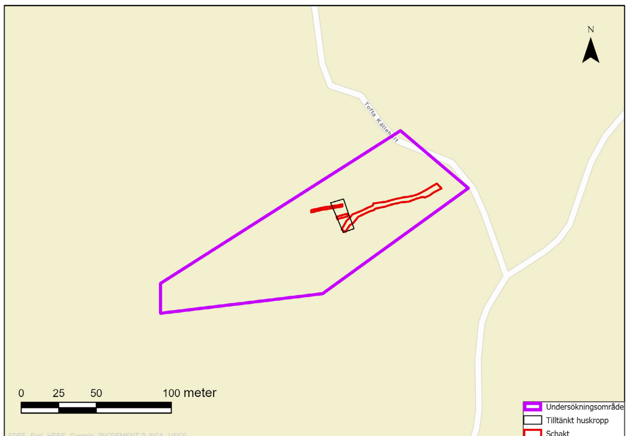
Figur 3. Plan över de schaktade ytorna inom undersökningsområdet som anpassades till de ingrepp som skulle ske.
